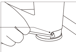
六角ネジ 固定ネジ拡大図
